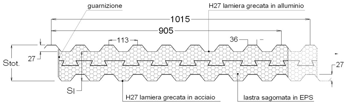
Sezione trasversale PANEL C-GG ST
