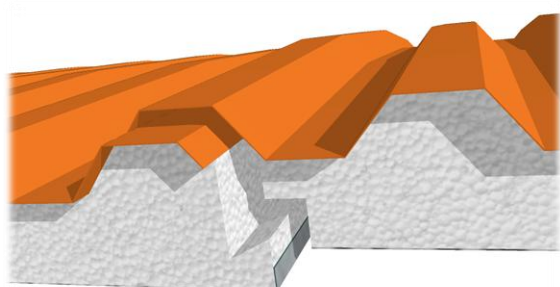
Particolare del giunto "anticondensa"
